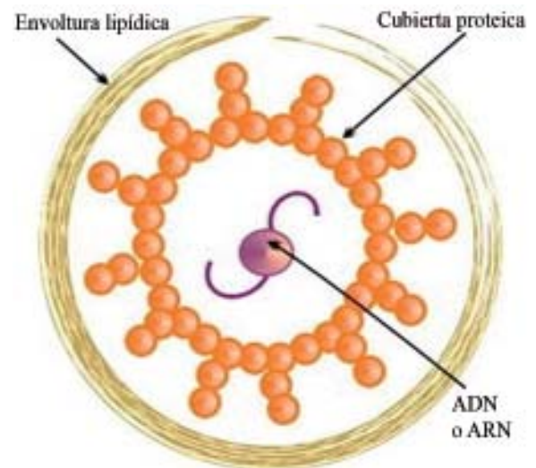
Fig. 25.2. Estructura viral.
