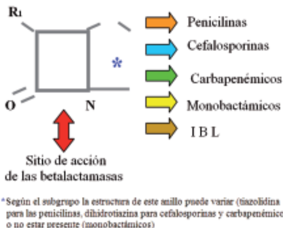
Fig. 23.4. Anillo betalactámico.
